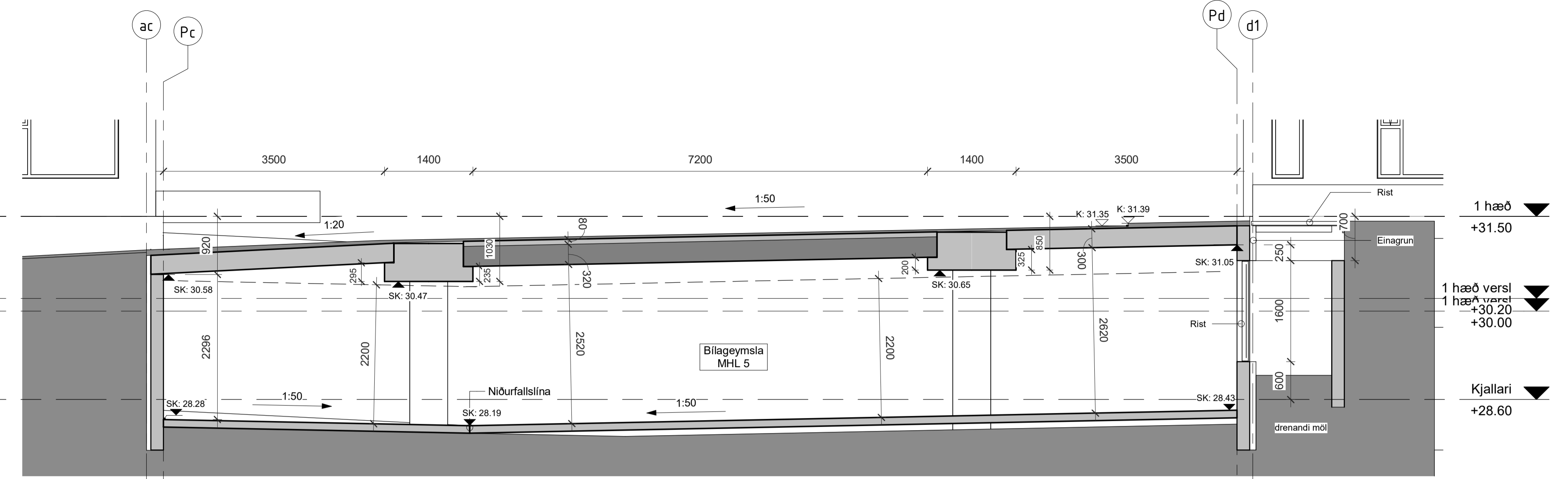
5A-Þversnið vesturenda 1 : 50
