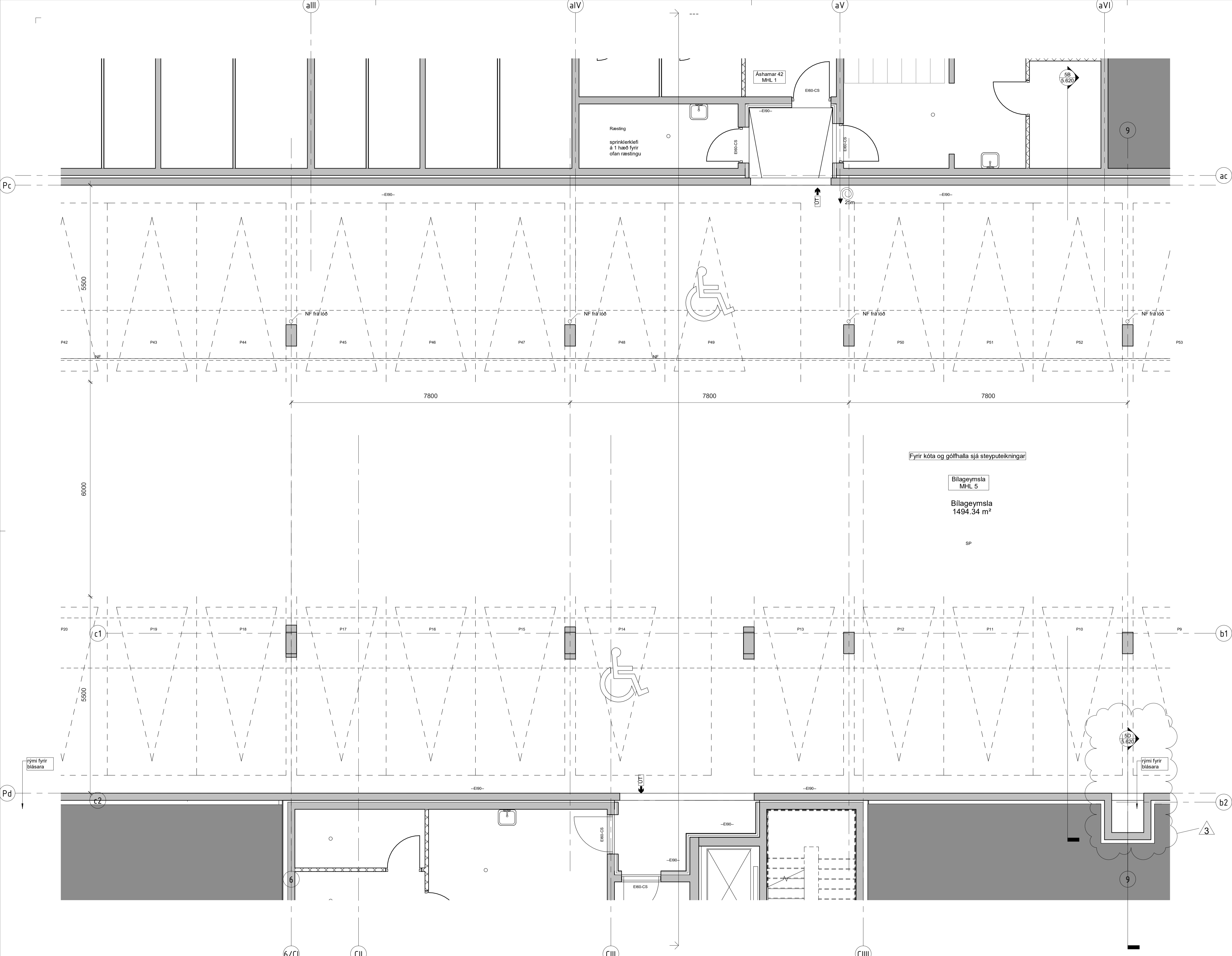
Kjallari vt - 2 1 : 50
