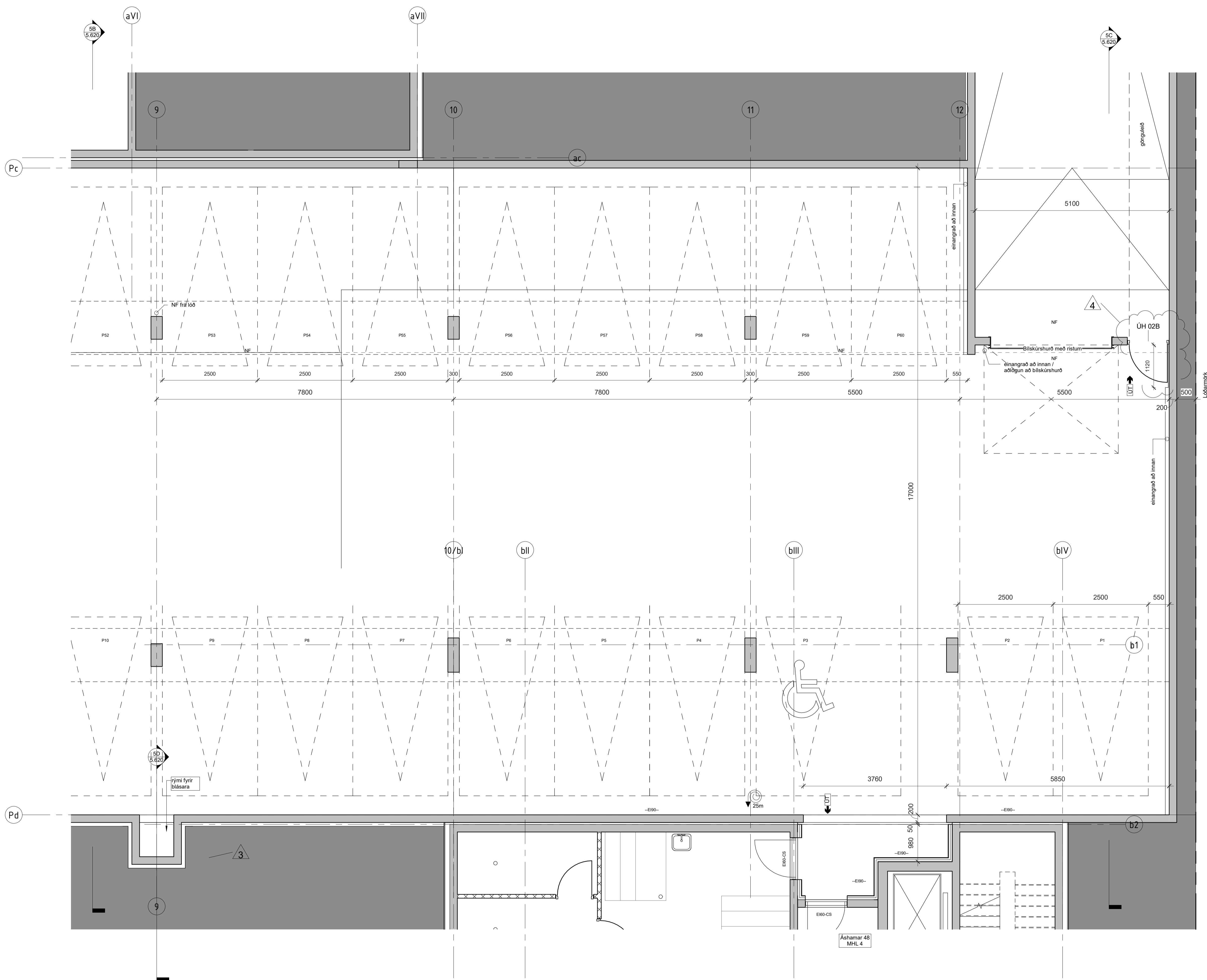
Kjallari vt - 3 1 : 50
